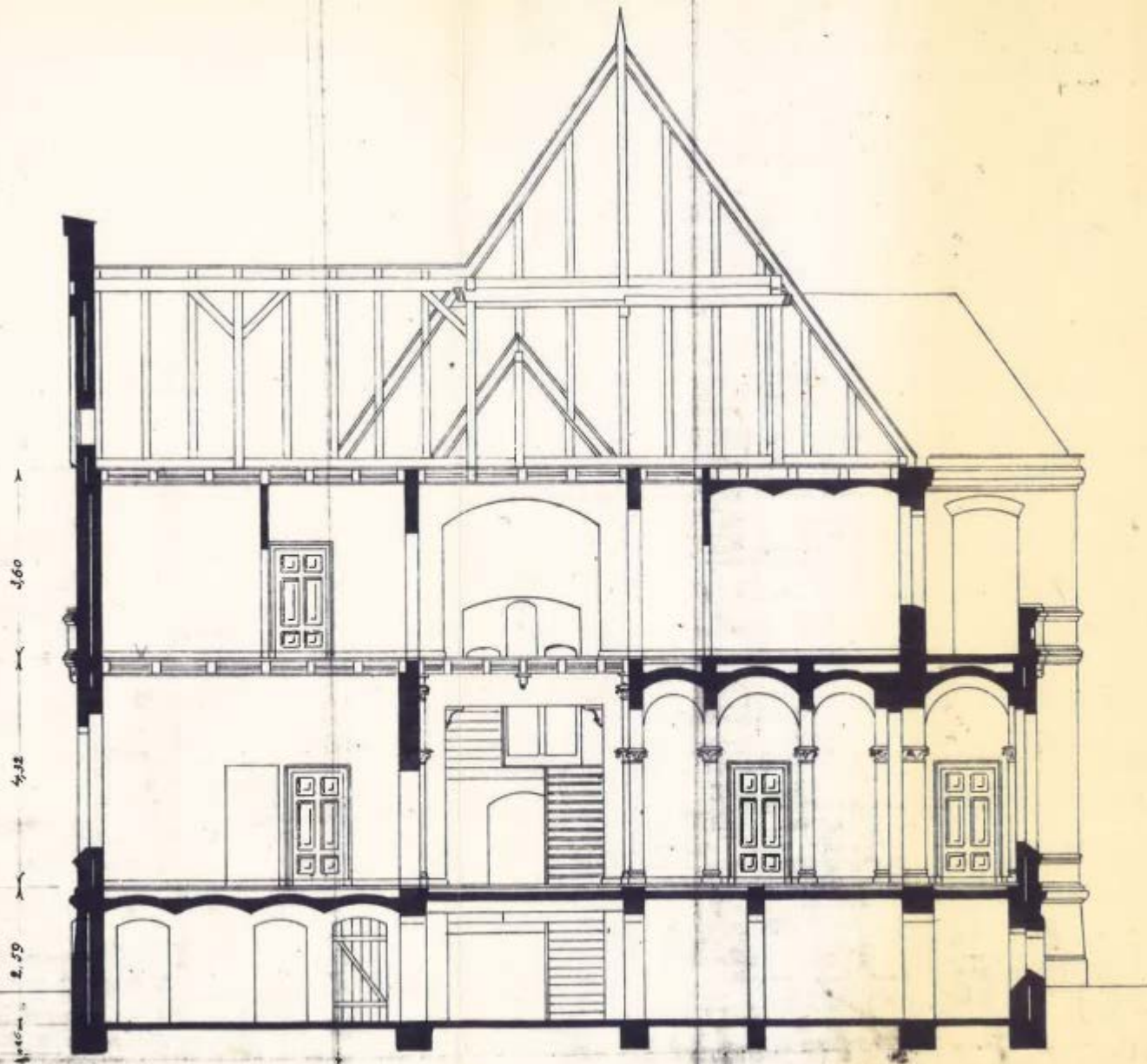
Querschnitt A-B.
